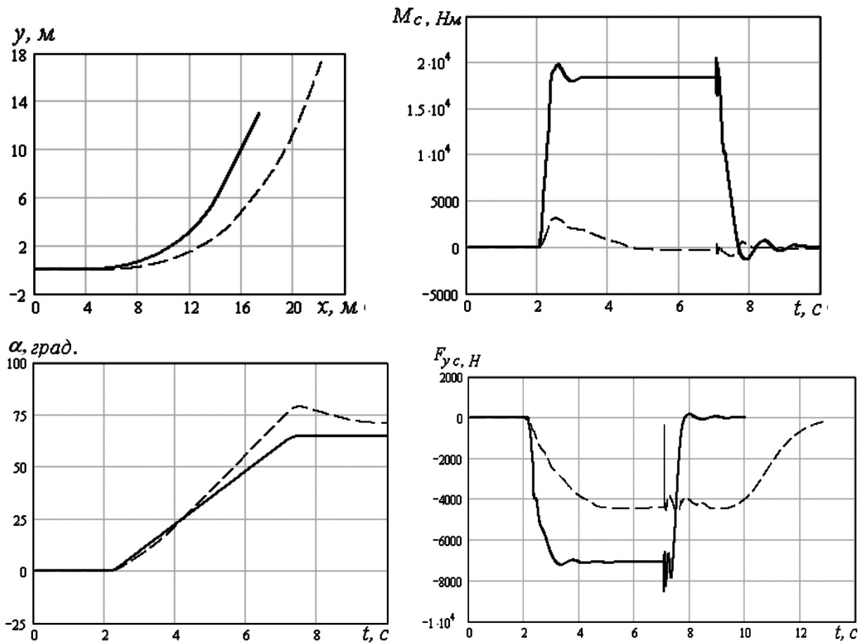
Рис.6.15. Динамические процессы при повороте машины.
