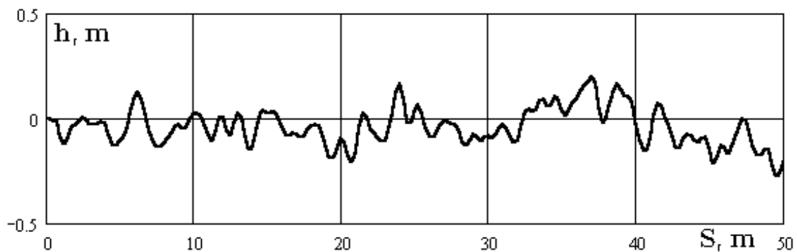
Рис. 6.21. Фрагмент микропрофиля трассы
