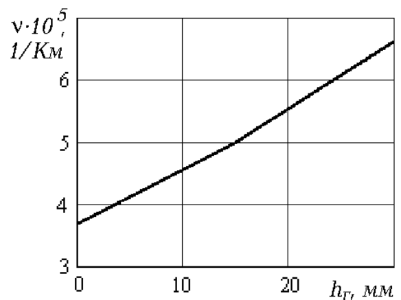
Рис.8.12. Влияние высоты гунтозацепов на удельное накопленное повреждение
