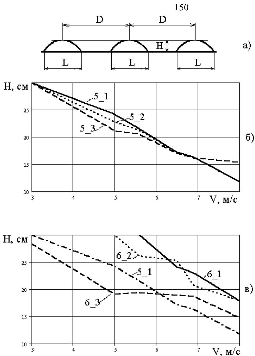
Рис.6.18. Функции быстроходности транспортной машины а)– стандартная низкочастотная трасса; б)– функция быстроходности для пятикаткового варианта машины ( 5_1– исходная подвеска, 5_2– сопротивление амортизаторов снижено на 25%, 5_3– на 50%); в)– функция быстроходности для шестикаткового варианта машины (6_1– исходная подвеска, 6_2– сопротивление амортизаторов снижено на 25%, 6_3–добавлен третий амортизатор)
