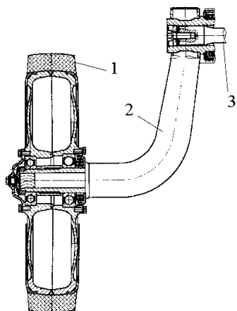
Рис.9.4. Элементы подвески снегоболотоходной машины: 1- опорный каток, 2- балансир, 3- торсион.
