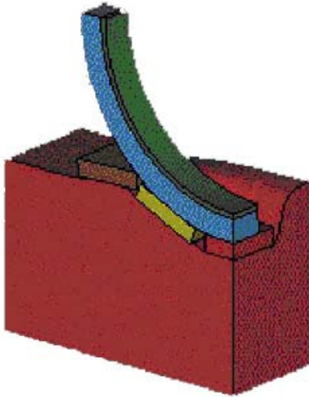
Рис. 4.14. Деформированное состояние грунта в активном участке
