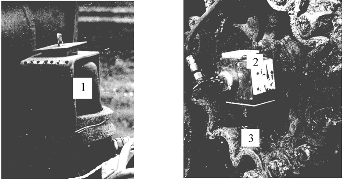
Рис.6.9. Установка измерительной аппаратуры. 1 – гироскоп, 2 – токосъемник
