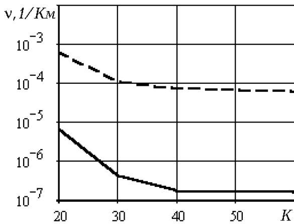
Рис.8.9. Зависимость удельного накопленного повреждения от предполагаемого числа точек контакта (1– c=20 \text{ МН/м}^3 , 2– c=50 \text{ МН/м}^3 )
