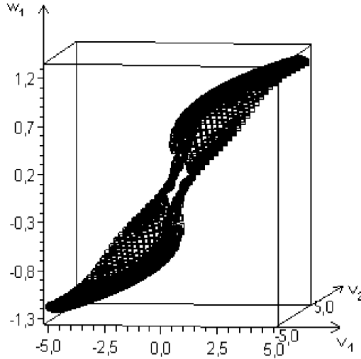
Рис.2 Проекция фазового пространства задачи (4)-(6) при \lambda = 1 , \delta = 1 , \beta = 1 , если
